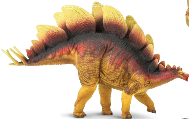
■ Stegosaurus (STEG-o-SORE-us)
